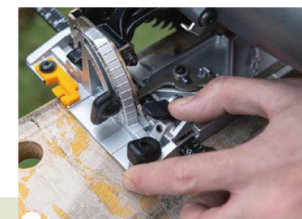
独自機構で平行定規の固定はワンタッチ。これは簡単!
