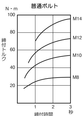
普通ボルト ボルト締付トルク
