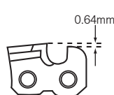
デプスゲージセッティング
