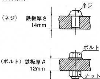
締付条件
