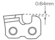
デプスゲージセッティング
