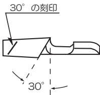
左刃目立て角度
