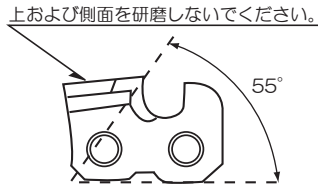
上刃切削角度
