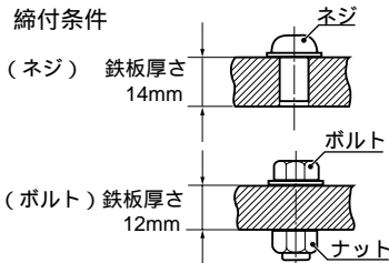
締付条件
