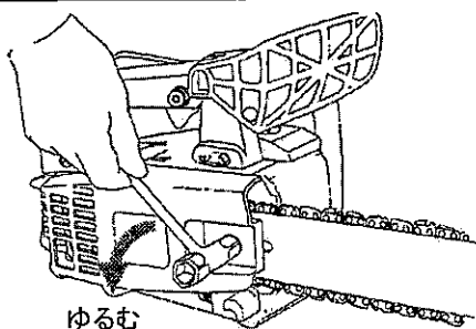
図16 ソーチェン
