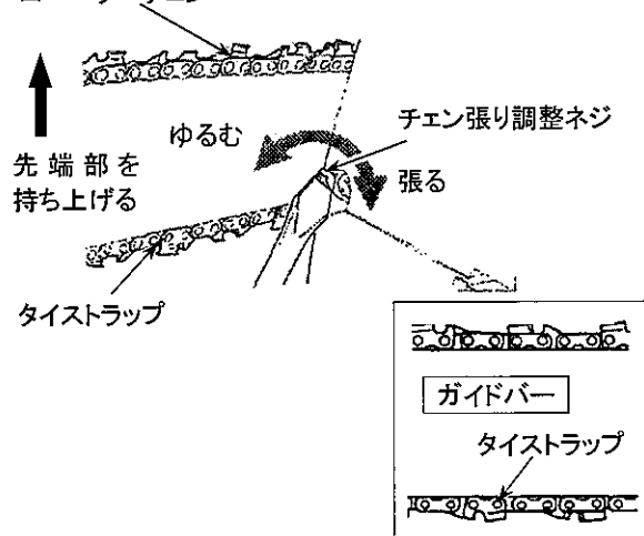
図16 ソーチェン
