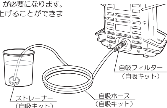
自吸キット
