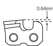
デブスゲージセッティング
