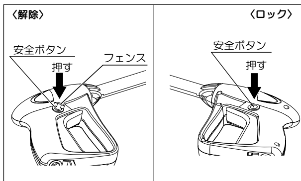
ガンを上から見た状態
