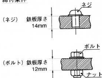
締付条件
