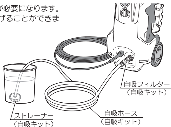
自吸キット
