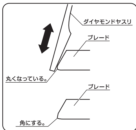
(ブレード側面部の断面図)
