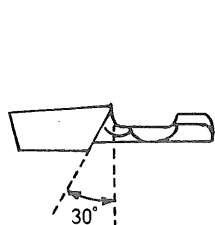
上刃目立角度
