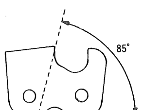
横刃目立角度
