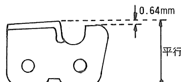
デプスゲージ
