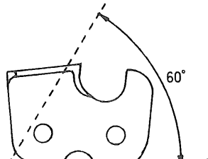
上刃切削角度
