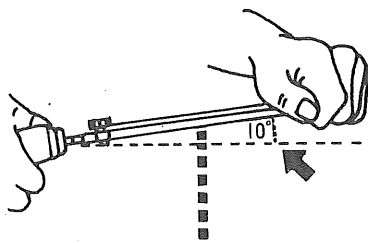
ヤスリの手前を10° 下げる
