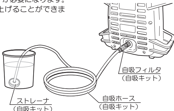
自吸キット
