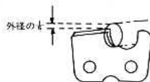
ヤスリの外径の1/5を上に出す。
