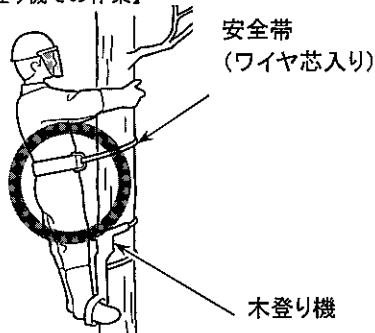
図18【木登り機での作業】
