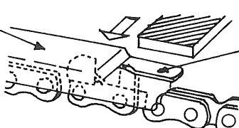
デプスゲージ ジョイント
