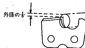
ヤスリの外径の1/5を上に出す。
