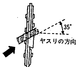
カッターの内側から外側に目立てる
