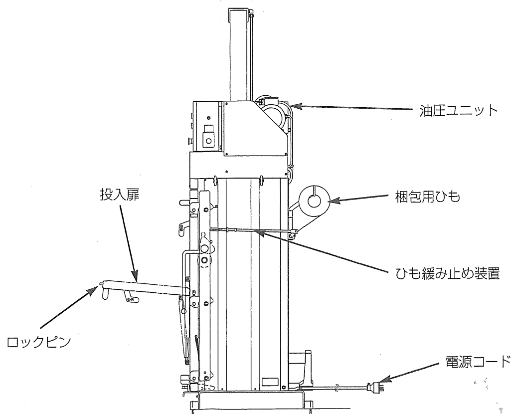
側面図
