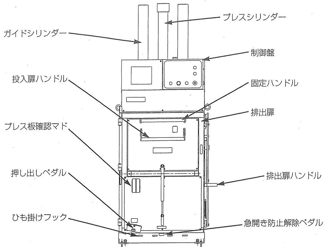
正面図
