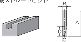
超硬ストレートビット
