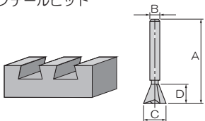
ダブルテールビット
