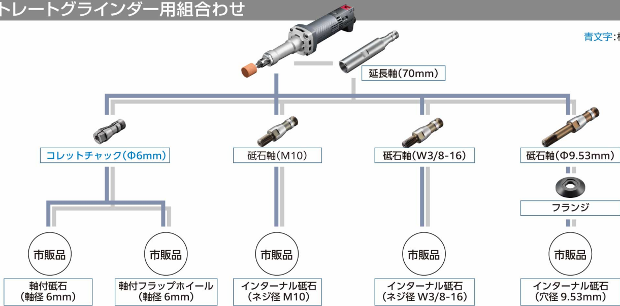
砥石軸
